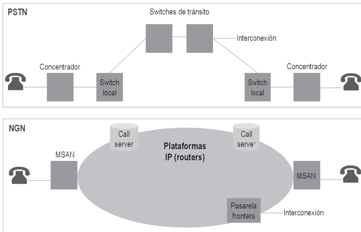
Figura 3. Comparación de la red PSTN tradicional y los servicios de voz sobre una NGN
