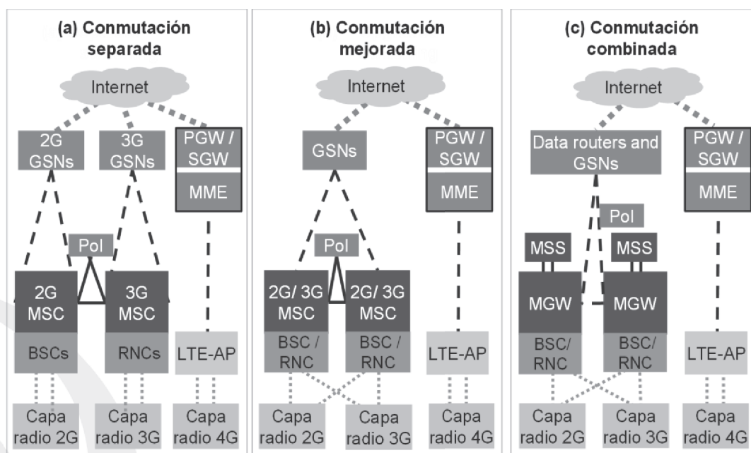
Figura 1. Opciones de arquitectura para el Modelo Móvil.
