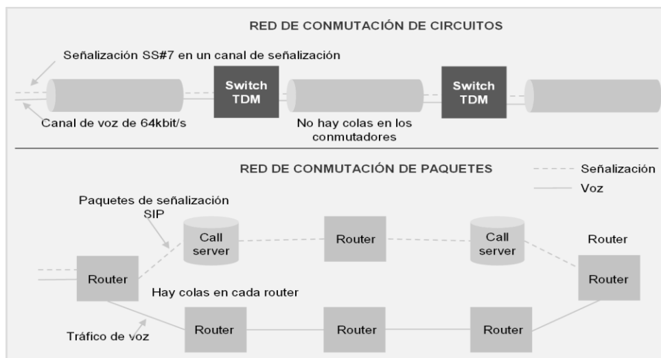
Figura 2. Comparación entre redes de conmutación de circuitos y de conmutación de paquetes
