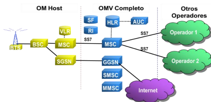
Diagrama 1. Elementos de la infraestructura de la red de un OMV Completo
