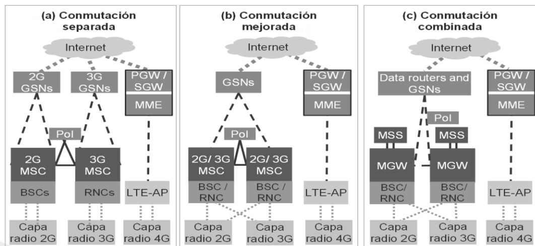
Figura 1. Opciones de arquitectura para el Modelo Móvil.
