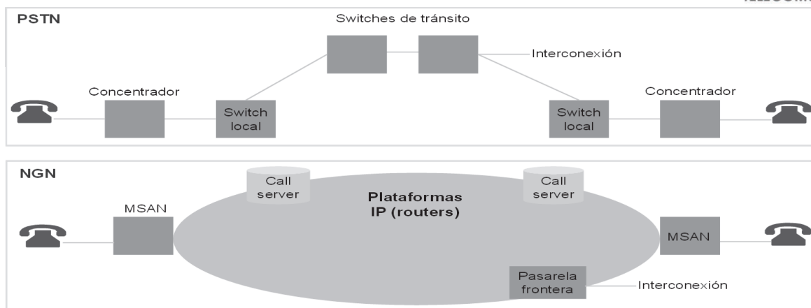
Figura 3. Comparación de la red PSTN tradicional y los servicios de voz sobre una NGN
