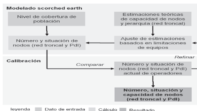
Figura 4. Esquema de modelado scorched-earth calibrado para el operador fijo
