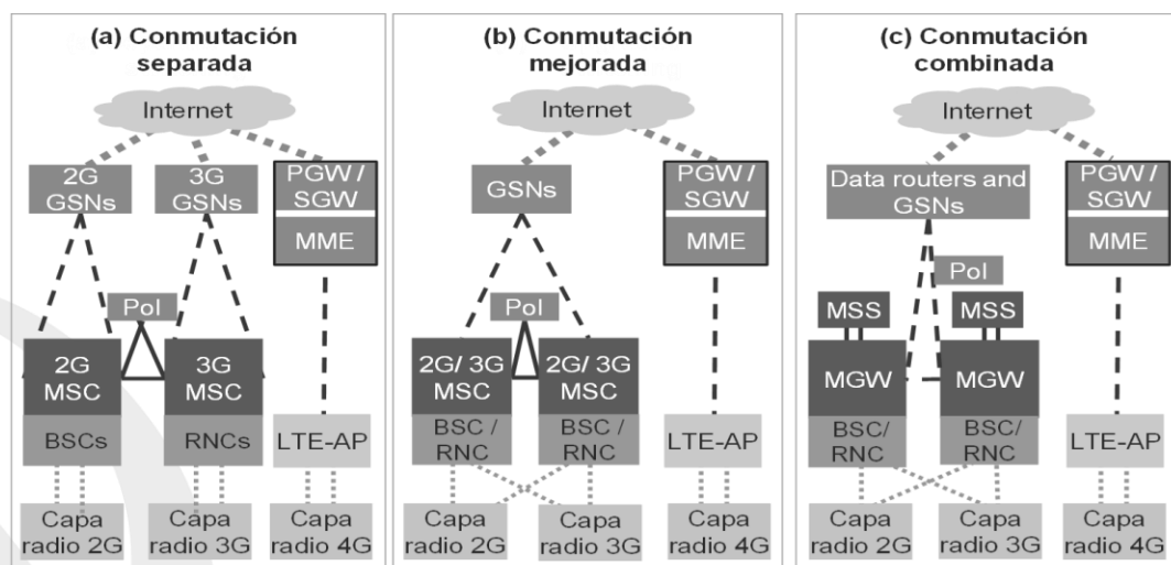
Figura 1. Opciones de arquitectura para el Modelo Móvil.
