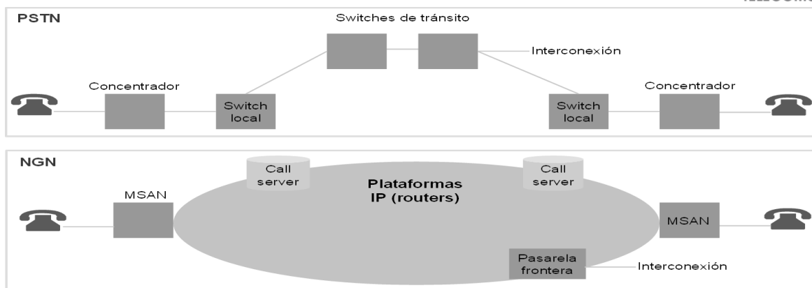
Figura 3. Comparación de la red PSTN tradicional y los servicios de voz sobre una NGN
