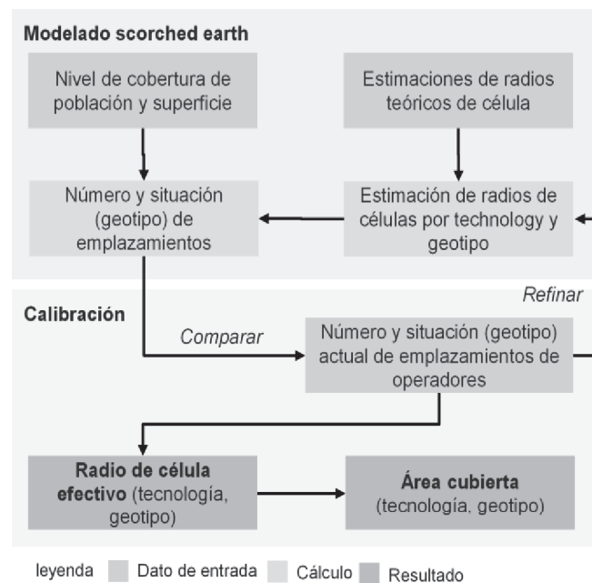
Figura 5. Esquema de modelado scorched earth calibrado para el operador móvil
