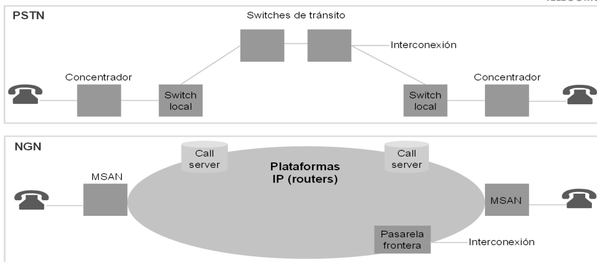
Figura 3. Comparación de la red PSTN tradicional y los servicios de voz sobre una NGN
