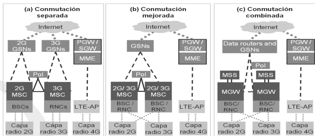
Figura 1. Opciones de arquitectura para el Modelo Móvil.
