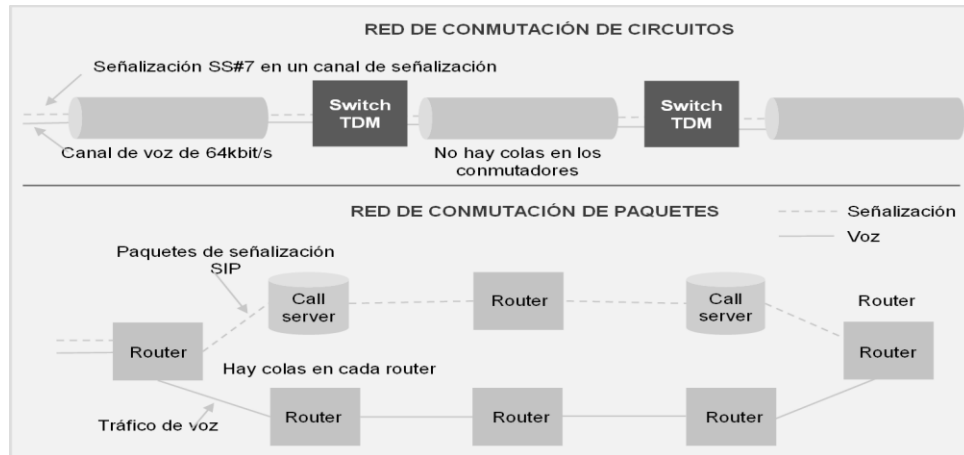
Figura 2. Comparación entre redes de conmutación de circuitos y de conmutación de paquetes
