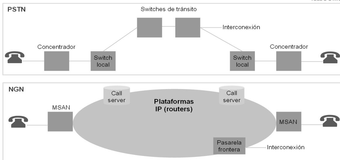
Figura 3. Comparación de la red PSTN tradicional y los servicios de voz sobre una NGN
