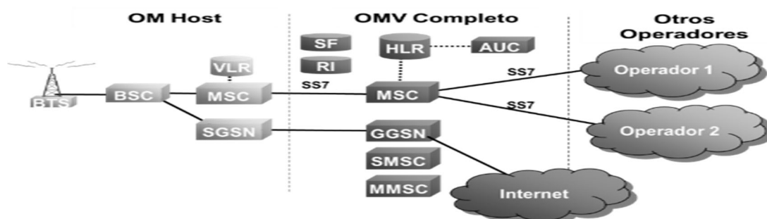
Diagrama 1. Elementos de la infraestructura de la red de un OMV Completo
