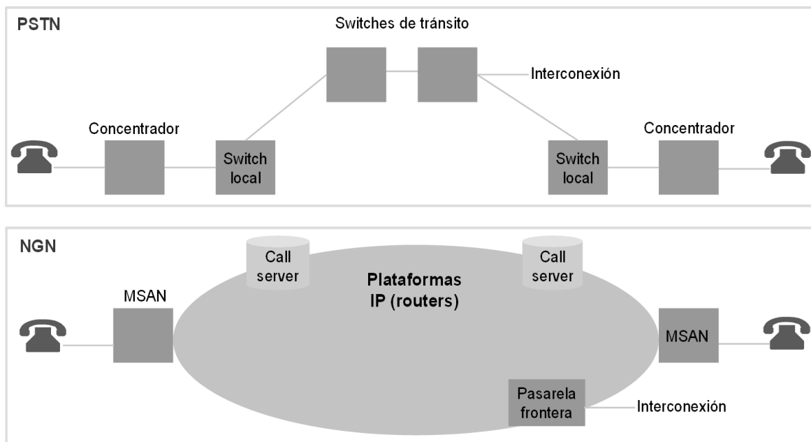
Figura 2. Comparación de la red PSTN tradicional y los servicios de voz sobre una NGN
