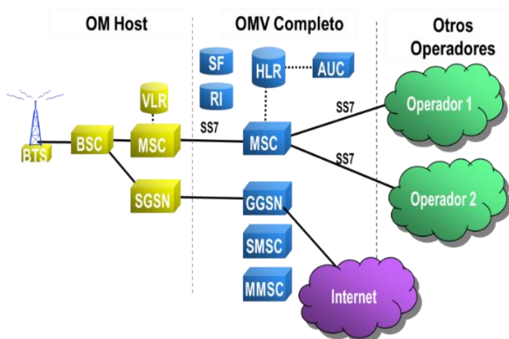
Diagrama 2. Elementos de la infraestructura de la red de un OMV Completo
