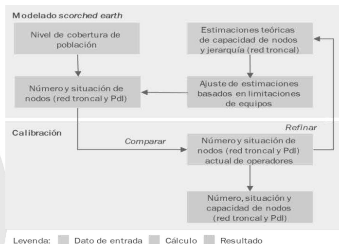
Figura 3. Esquema de modelado scorched-earth calibrado para el operador fijo
