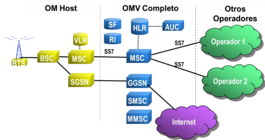
Diagrama 2. Elementos de la infraestructura de la red de un OMV Completo
