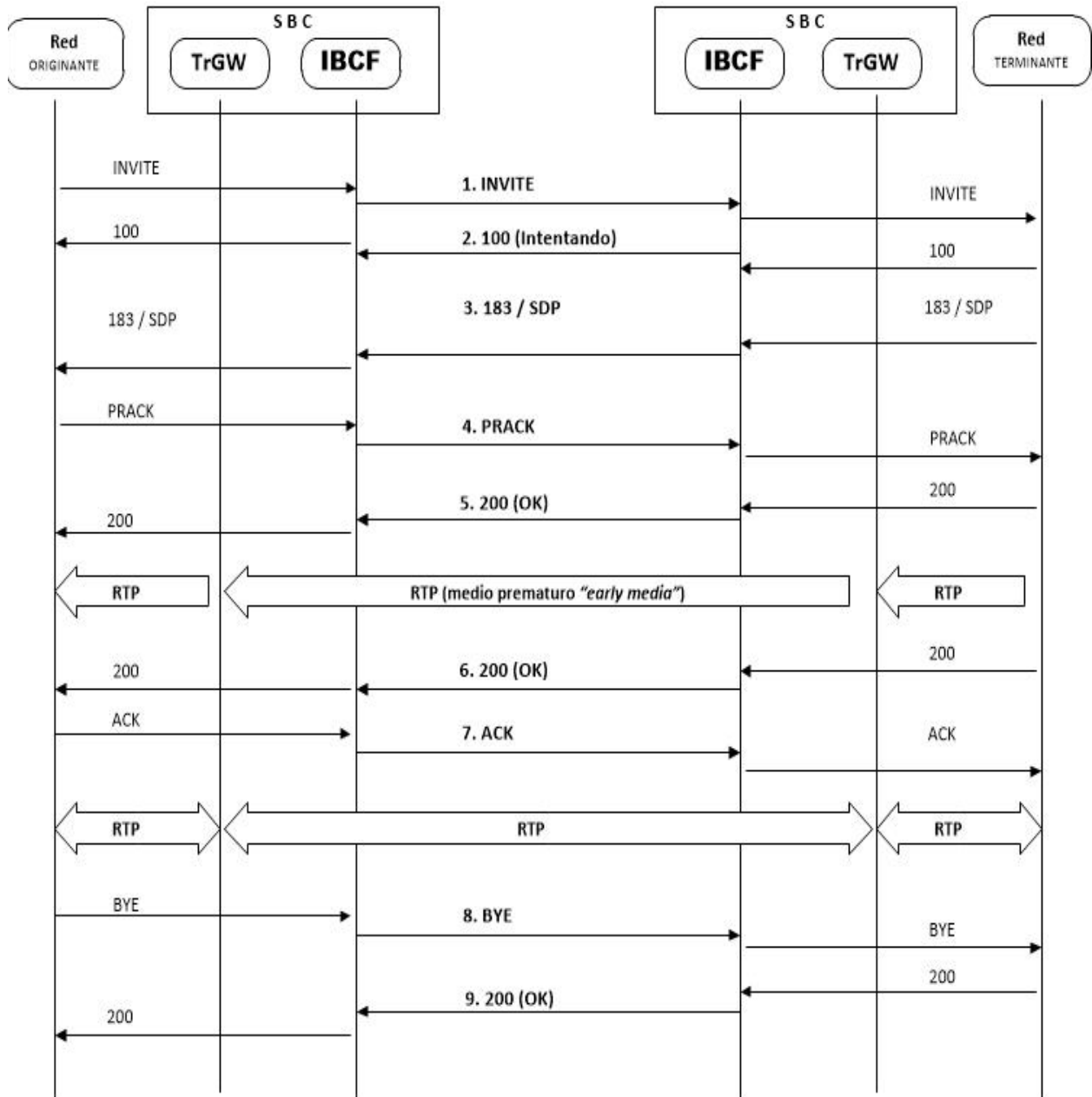
Diagrama 2. Establecimiento de una llamada básica con medio temprano.
