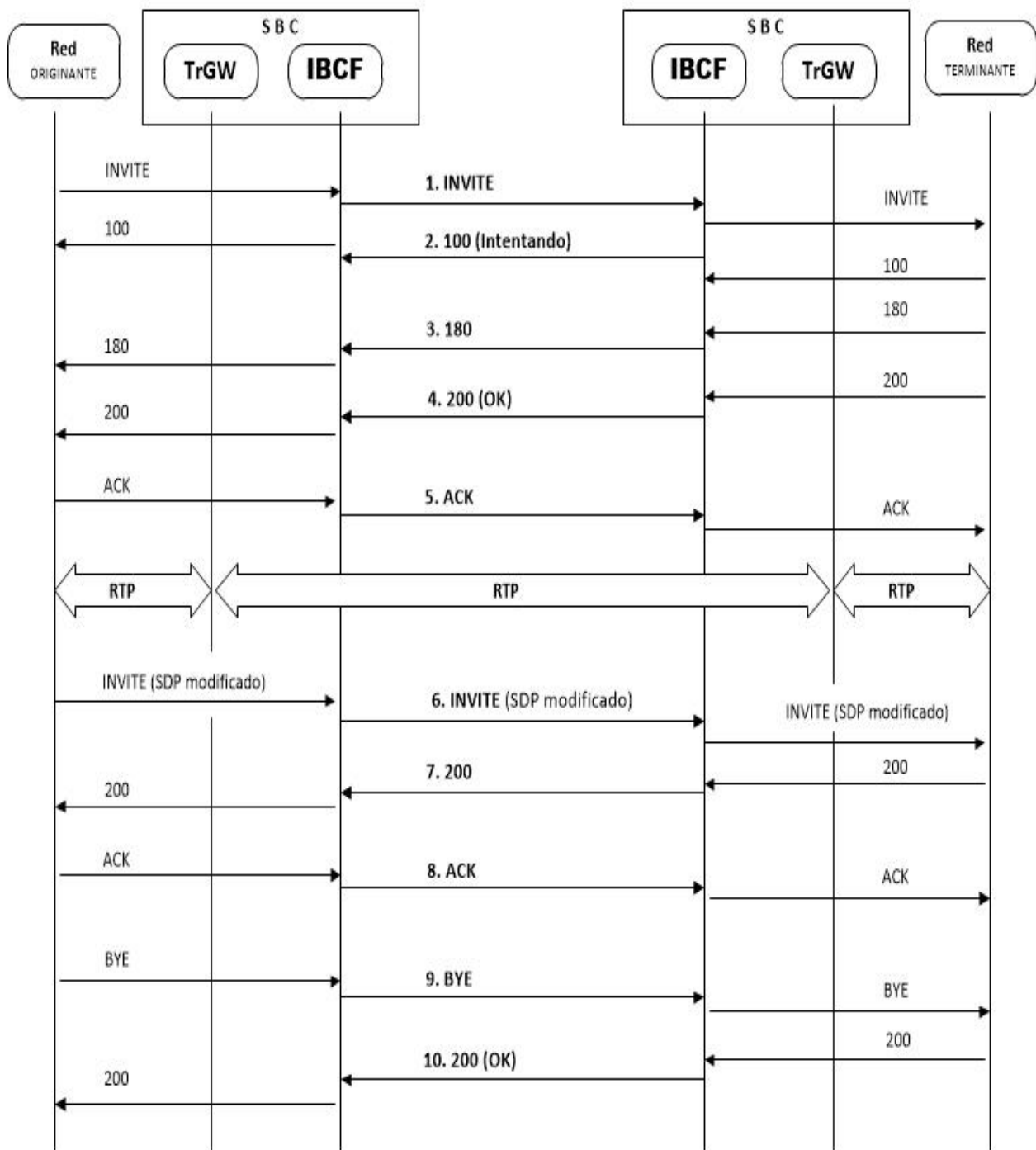
Diagrama 4. Actualización del medio.
