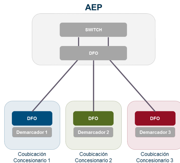
Fig. 2. Arquitectura servicio de interconexión cruzada activo.
