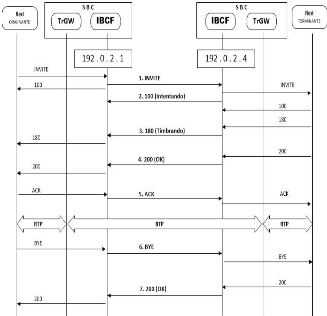
Diagrama 1. Establecimiento de una llamada básica.
