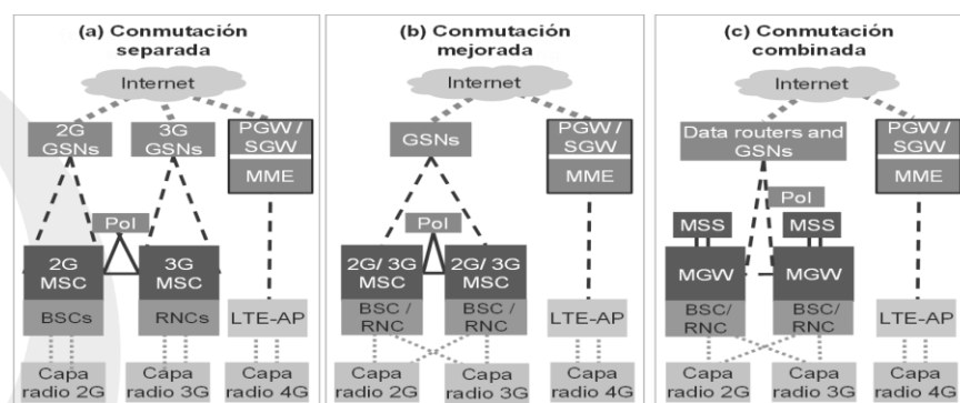
Figura 1. Opciones de arquitectura para el Modelo Móvil.
