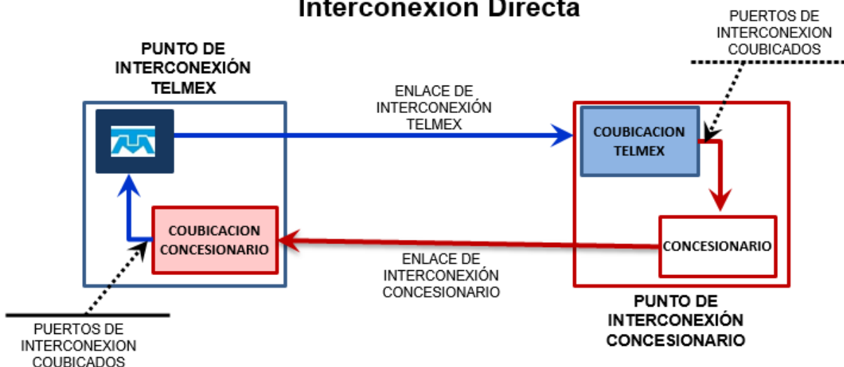
Diagrama de Interconexión para señalización SIP
