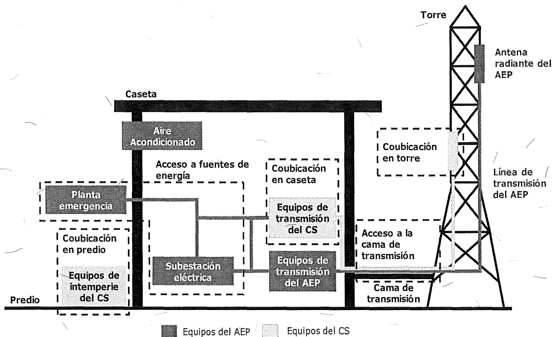
Figura 3: Servicios de coubicación (Fuente: IFT, 2019)
