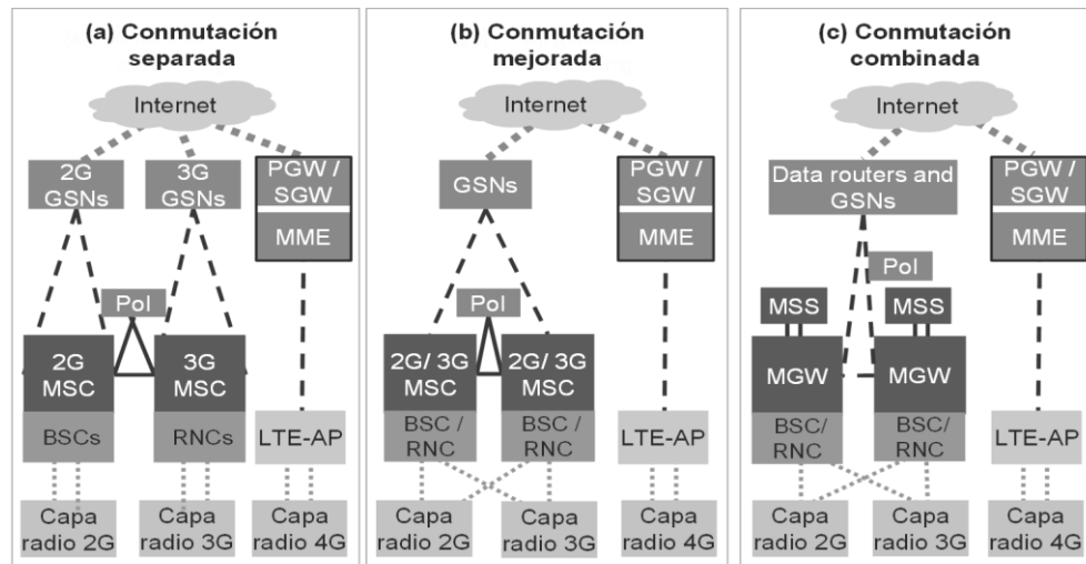
Figura 1. Opciones de arquitectura para el Modelo Móvil.
