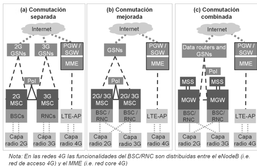
Figura 1. Opciones de arquitectura para el Modelo Móvil.
