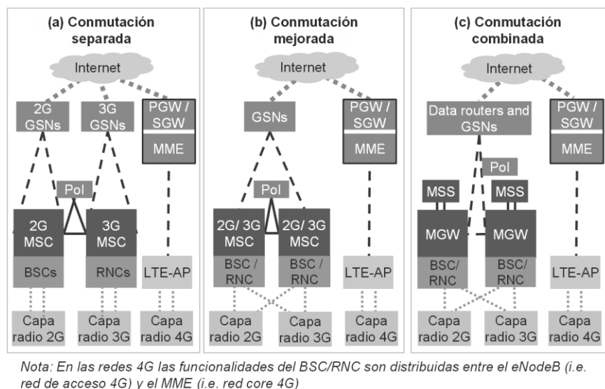
Figura 1. Opciones de arquitectura para el Modelo Móvil.
