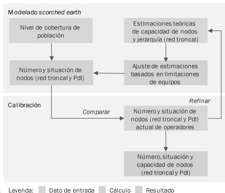
Figura 3. Esquema de modelado scorched-earth calibrado para el operador fijo
