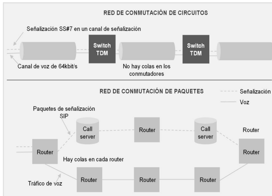
Figura 1. Comparación entre redes de conmutación de circuitos y de conmutación de paquetes
