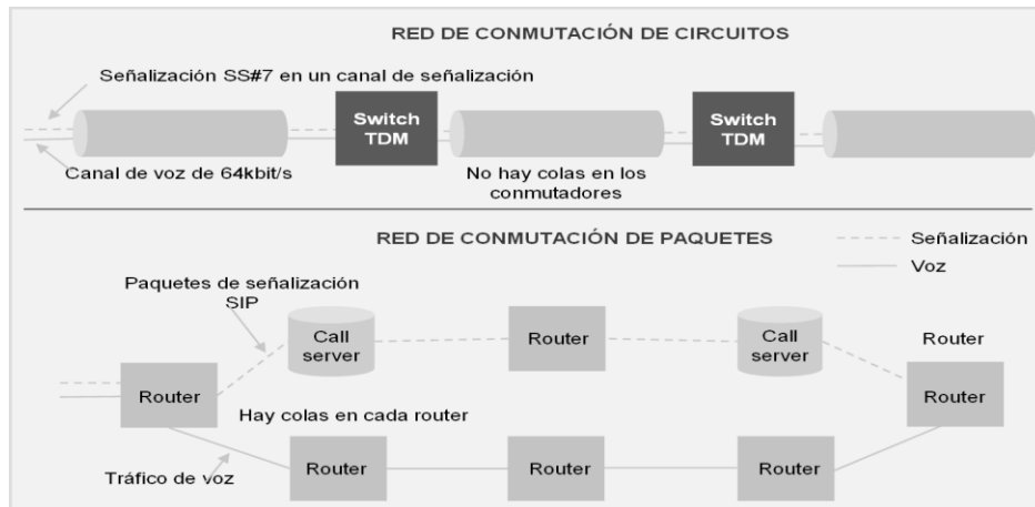
Figura 1. Comparación entre redes de conmutación de circuitos y de conmutación de paquetes
