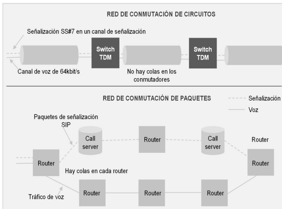
Figura 1. Comparación entre redes de conmutación de circuitos y de conmutación de paquetes
