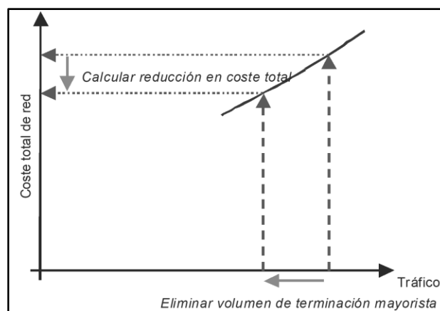
Figura 7. Cálculo del costo incremental del tráfico de terminación.
