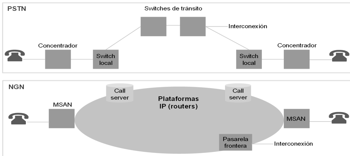
Figura 2. Comparación de la red PSTN tradicional y los servicios de voz sobre una NGN
