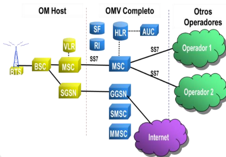
Diagrama 2. Elementos de la infraestructura de la red de un OMV Completo
