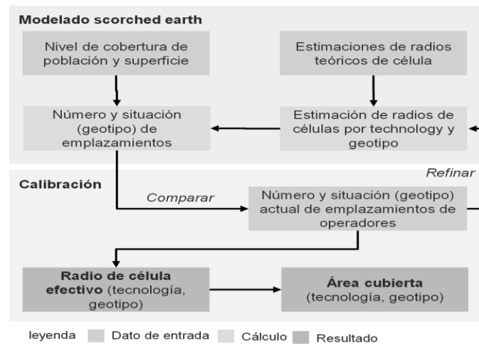
Figura 4. Esquema de modelado scorched earth calibrado para el operador móvil
