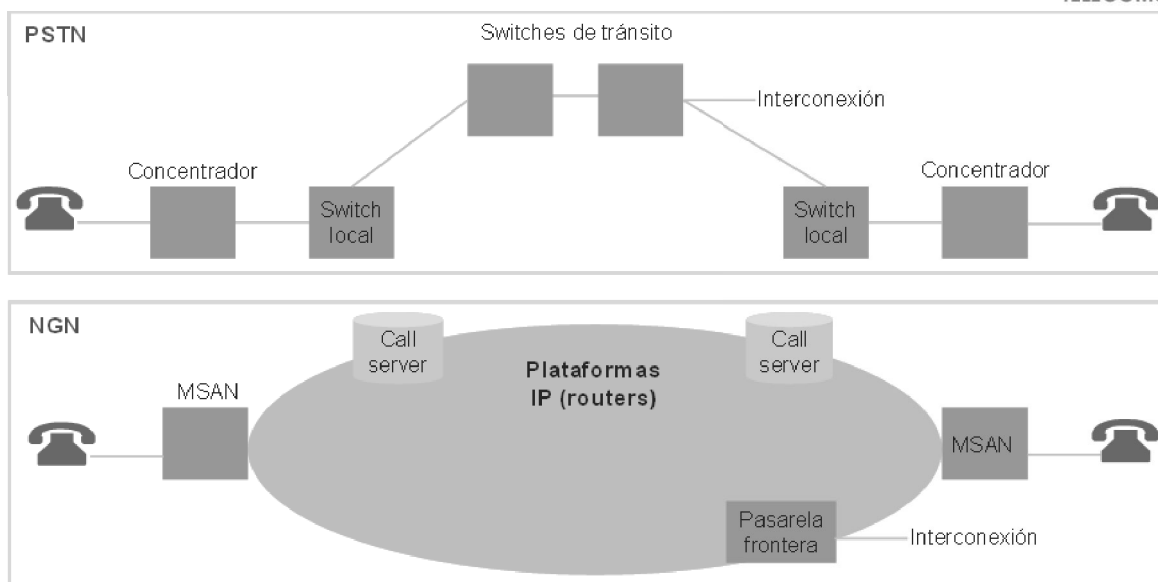
Figura 2. Comparación de la red PSTN tradicional y los servicios de voz sobre una NGN
