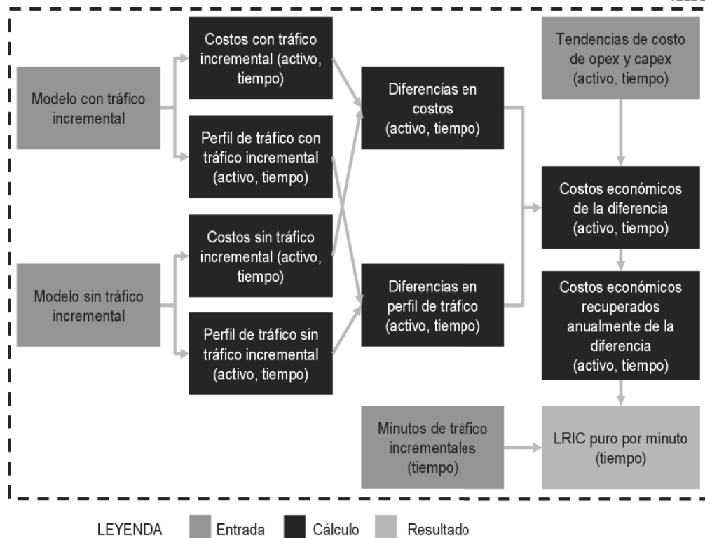
Figura 8. Etapas necesarias para el cálculo del CILP Puro.
