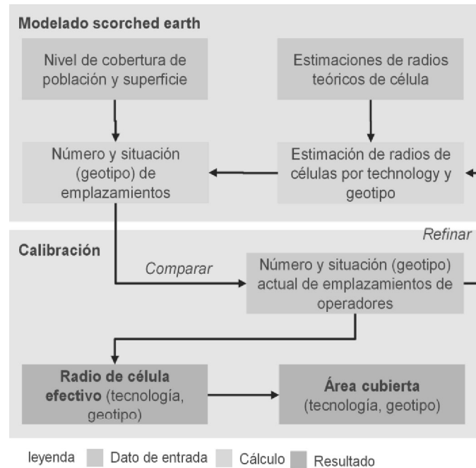
Figura 4. Esquema de modelado scorched earth calibrado para el operador móvil
