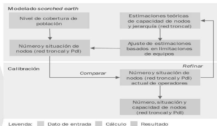
Figura 3. Esquema de modelado scorched-earth calibrado para el operador fijo
