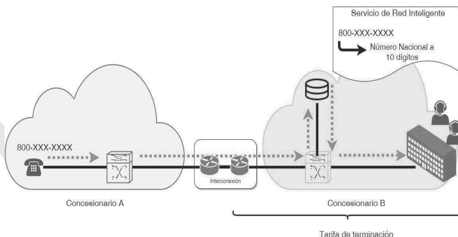
Diagrama 1. Las llamadas originadas en la red del Concesionario A con destino a un número 800 del Concesionario B son llamadas locales.
