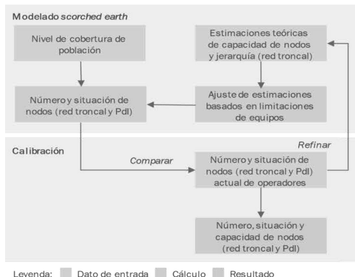
Figura 3. Esquema de modelado scorched-earth calibrado para el operador fijo
