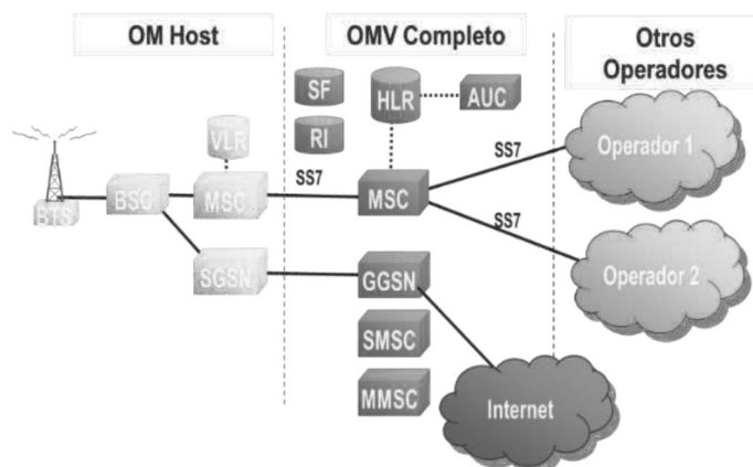
Diagrama 2. Elementos de la infraestructura de la red de un OMV Completo
