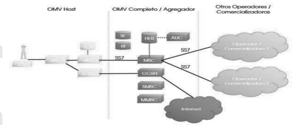
Diagrama 2. Elementos de la infraestructura de la red de un OMV Completo/Agregador
