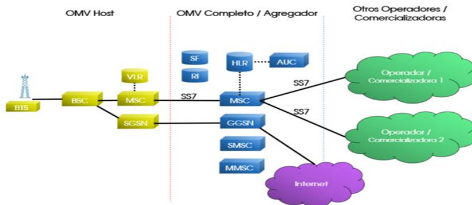
Diagrama 2. Elementos de la infraestructura de la red de un OMV Completo/Agregador
