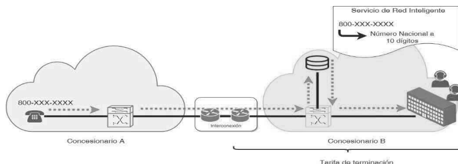
Diagrama 1. Las llamadas originadas en la red del Concesionario A con destino a un número 800 del Concesionario B son llamadas locales.
