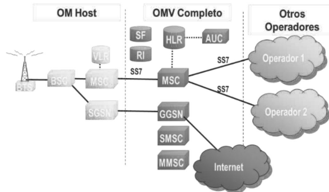
Diagrama 2. Elementos de la infraestructura de la red de un OMV Completo
