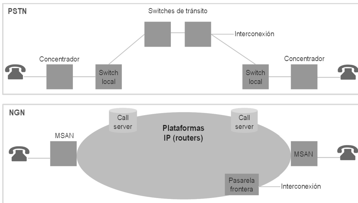
Figura 2. Comparación de la red PSTN tradicional y los servicios de voz sobre una NGN
