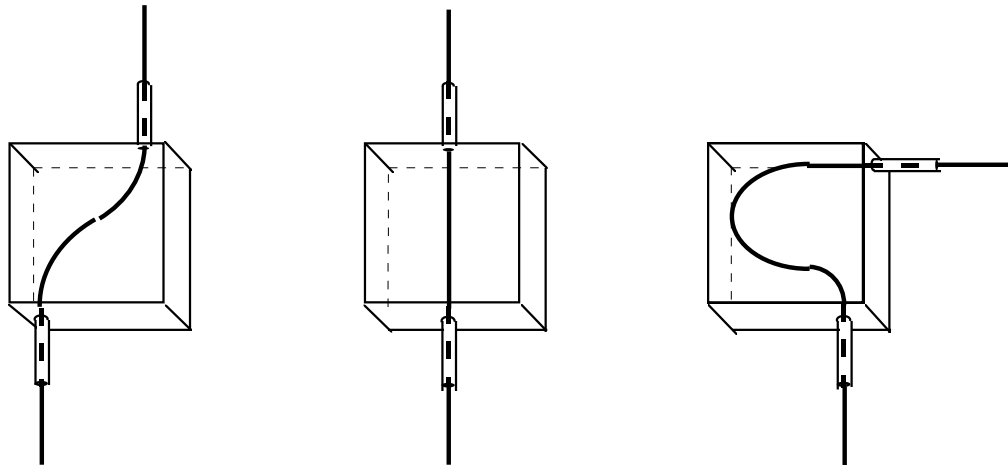
Colocación incorrecta de registros para Fibra óptica.
