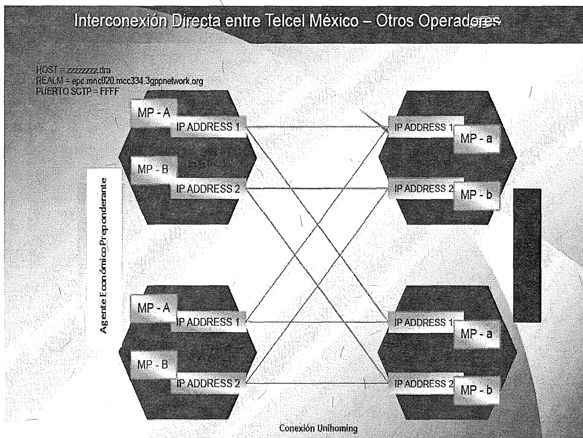
Figura 3: Diagrama de interconexión directa e indirecta vía señalización Diameter mediante interfaz S6a.
