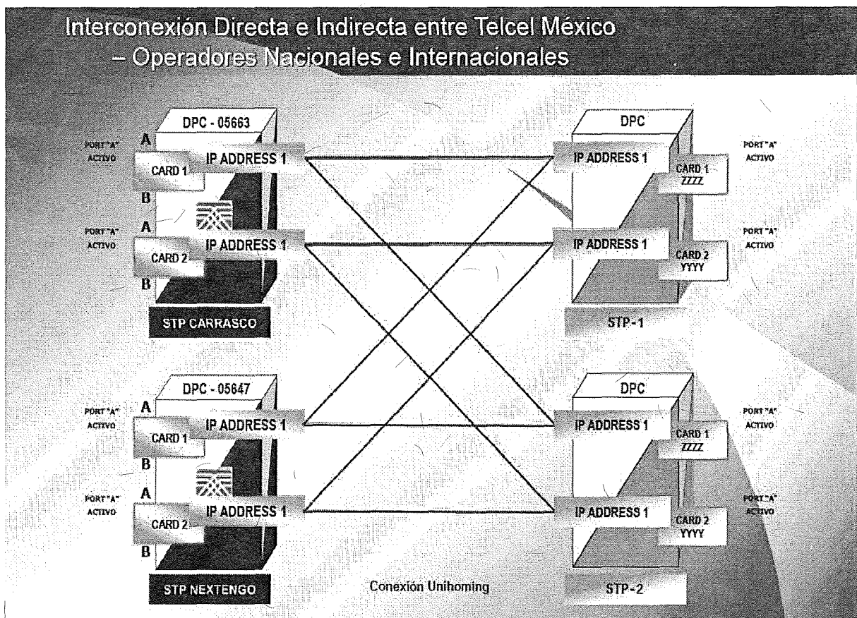
Figura 1: Topología requerida de interconexión de señalización con enlaces SIGTRAN M2PA entre Telcel y el Concesionario.
