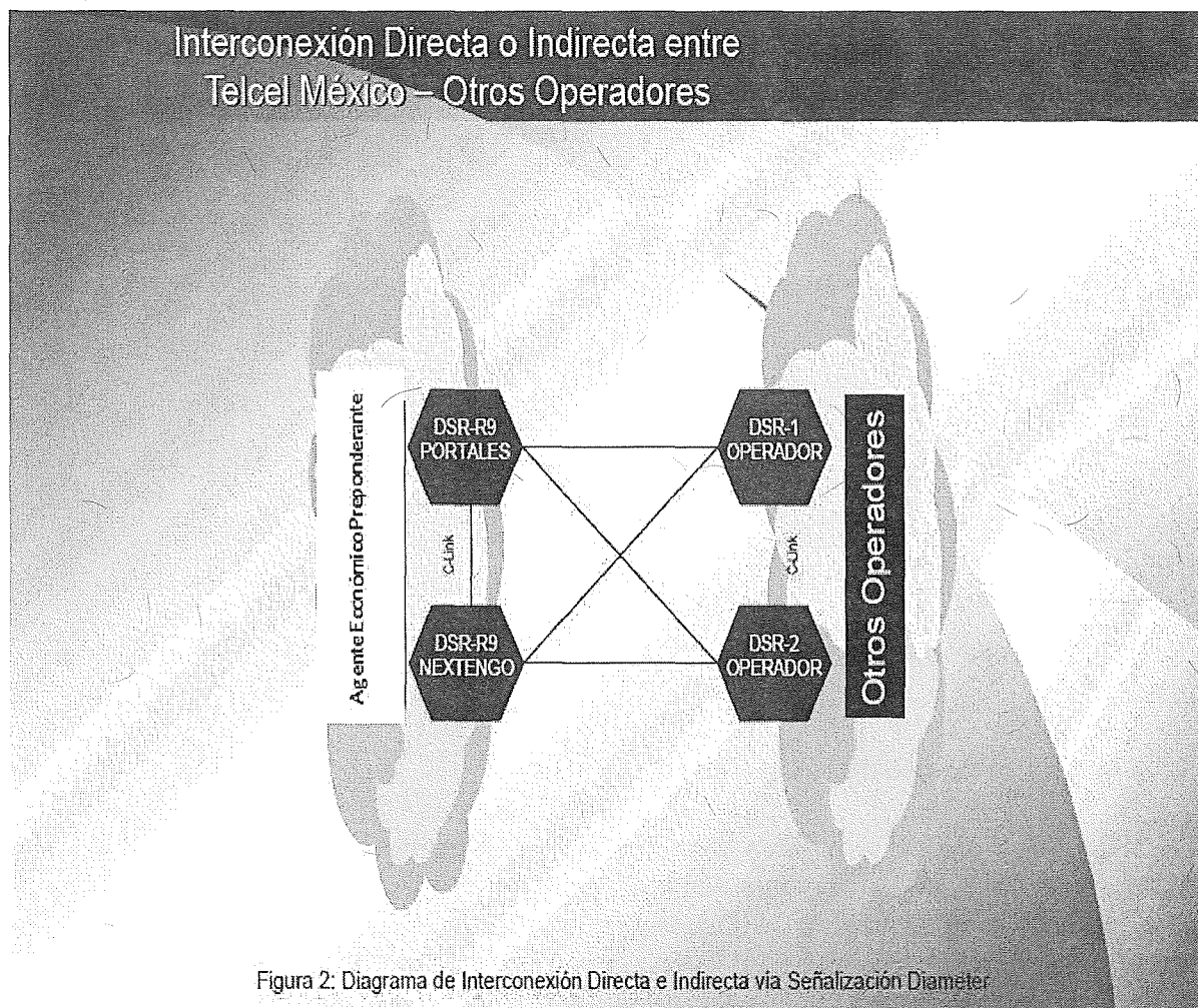
Figura 2: Diagrama de interconexión directa e indirecta vía señalización Diameter
