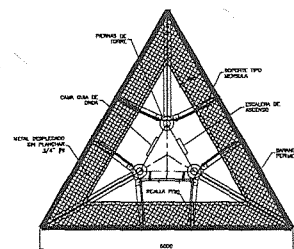
PLATAFORMA TRIANGULAR CELULAR DE 5m
