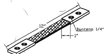
CONECTOR DE COBRE TRENZADO FLEXIBLE TIPO BD
