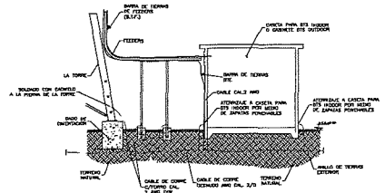
ATERRIJAJE DE ESTRUCTURAS METÁLICAS Y CONTENEDOR
