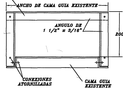
ALTERNATIVA PARA INTALACION DE CAMA GUIA GSM SOBRE CAMA EXISTENTE (ALZADO) SOPORTE TIPO PORTERIA
