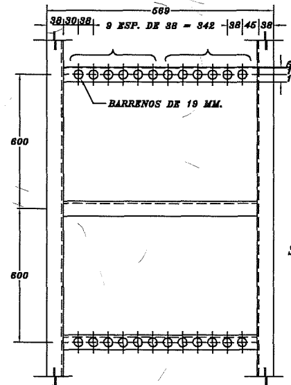
CAMA GUIA DE 12 BARRENOS (PLANTA)
