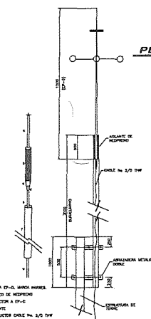
PLATAFORMA TRIANGULAR CELULAR DE 5m
