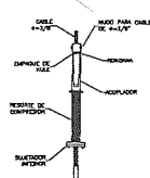
DETALLE B
