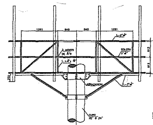
ELEVACION
