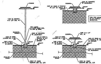
SOPORTE PARA CGO HORIZONTAL
