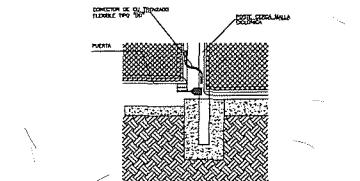
DETALLE DE ATERRIJAJE DE PUERTA DE MALLA CICLÓNICA
