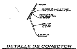
DETALLE DE CONECTOR
