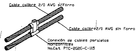
SOLDADURA CADWELD TIPO PT
