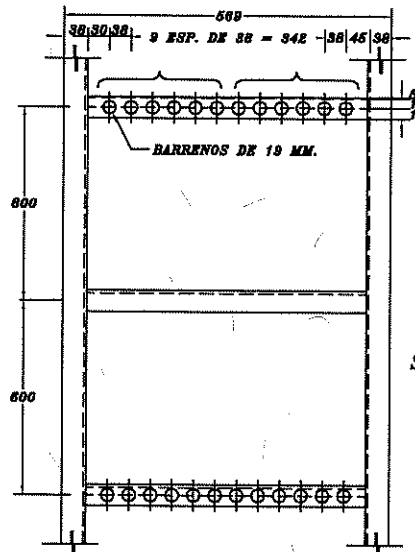
CAMA GUIA DE 12 BARRENOS (PLANTA)
