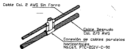
SOLDADURA CADWELD TIPO PT
