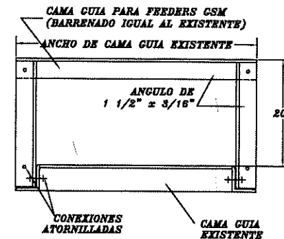
ALTERNATIVA PARA INTALACION DE CAMA GUIA GSM SOBRE CAMA EXISTENTE (ALZADO) SOPORTE TIPO PORTERIA
