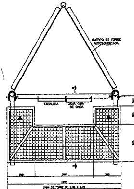
PLATAFORMA DE DESCANSO
