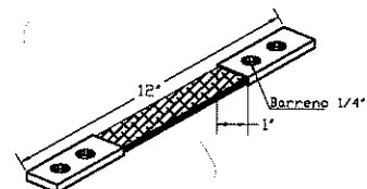
CONECTOR DE COBRE TRENZADO FLEXIBLE TIPO BD
