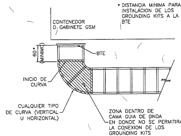
INSTALACION DE GROUNDING KITS
