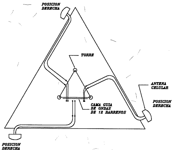
CRITERIOS DE DISTRIBUCION DE FEEDERS EN PLATAFORMAS
