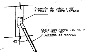
SOLDADURA CADWELD TIPO VS
