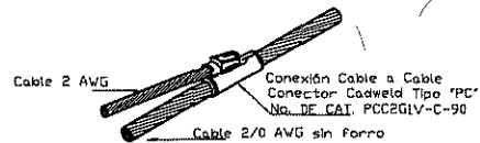
SOLDADURA CADWELD TIPO PC
