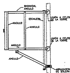
VISTA A'-A'
