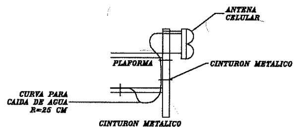
FIJACION DE FEEDERS Y JUMPER EN PLATAFORMA
