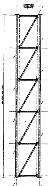
TRAMO DE TORRE ARRIOSTRADA
