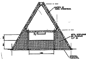
PLATAFORMA DE DESCANSO
