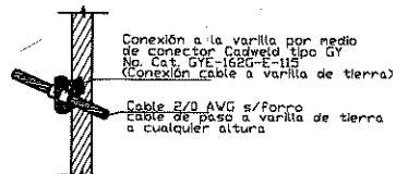
SOLDADURA CADWELD TIPO GY
