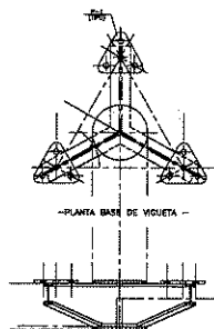
PLANTA BASE DE VIGUETA
