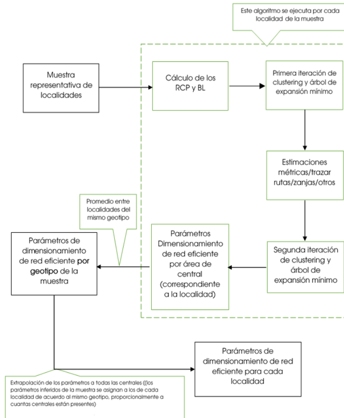
Figura 1: Esquema de los algoritmos de dimensionamiento de la red por geotipo.
