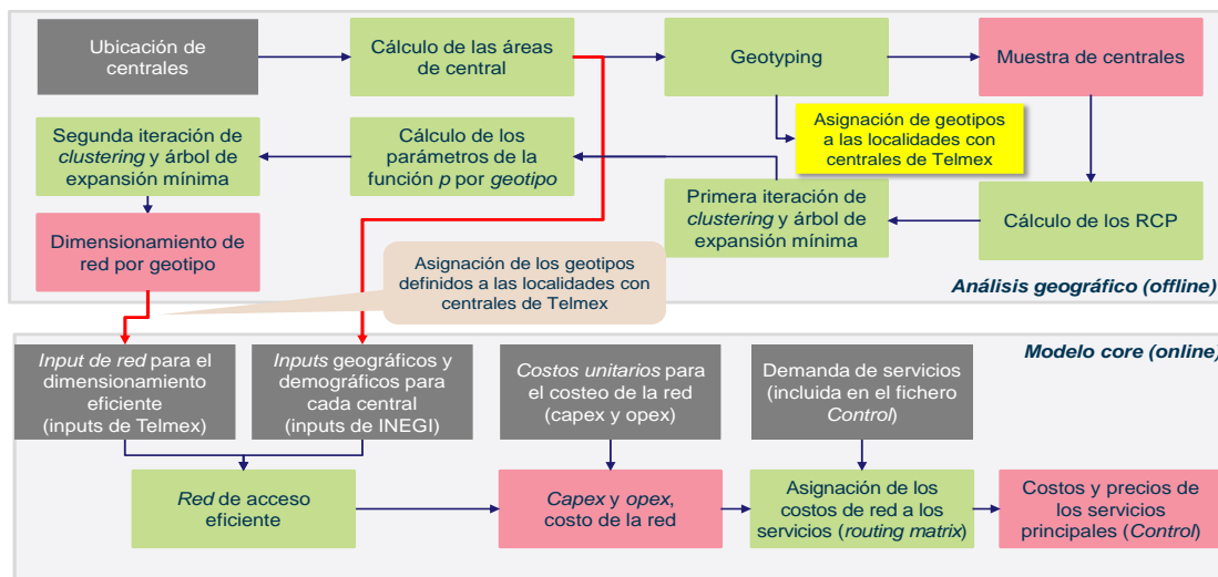
Figura 4: Diagrama de flujo del Modelo de Red de Acceso Fijo.
