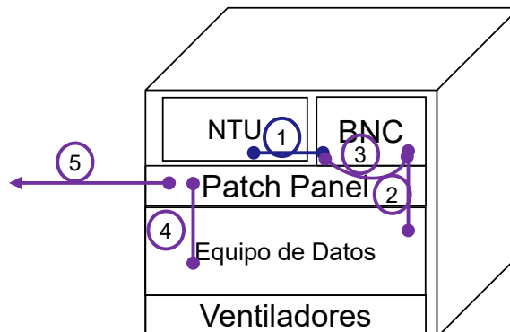
Responsabilidad de cableados en GUT y MIDI-GUT
