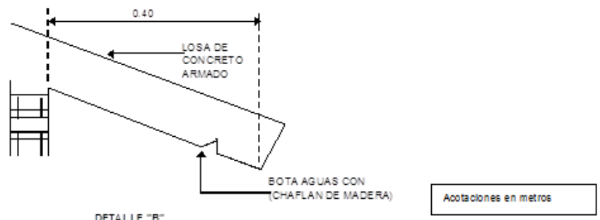
DETALLE "B"
