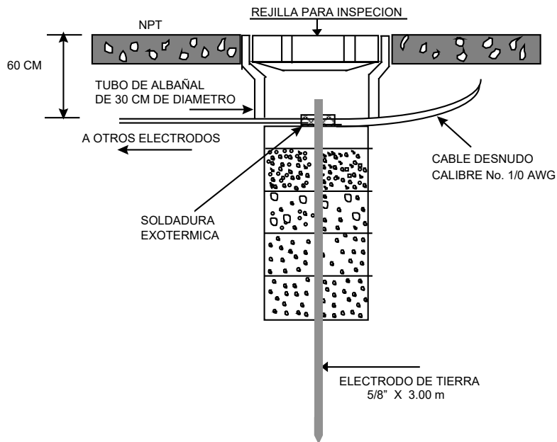
Registro de un Electrodo Copperweld
