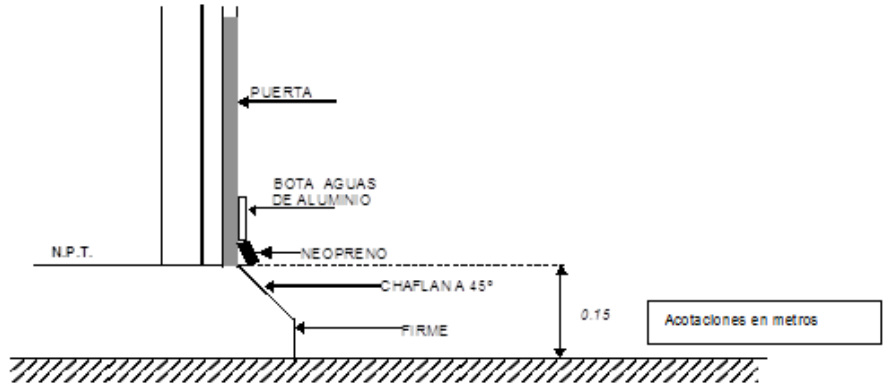
DETALLE "A"
