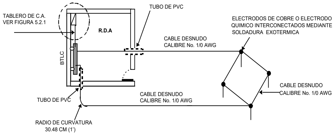
Puesta a Tierra del sitio cliente.
