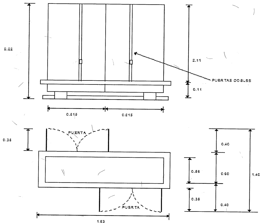
Dimensiones de equipo para edificio multicliente suministrado por La Empresa Mayorista.
