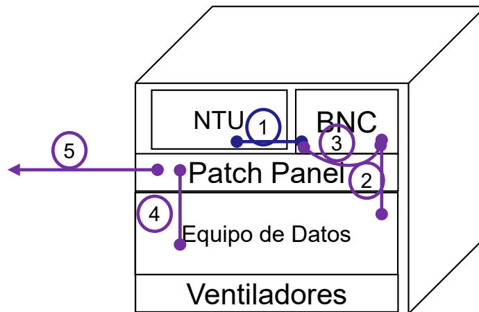
Responsabilidad de cableados en GUT y MIDI-GUT
