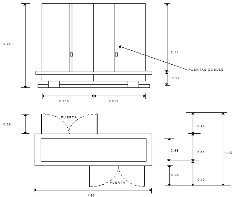
Dimensiones de equipo para edificio multicliente suministrado por División Mayorista Telmex.
