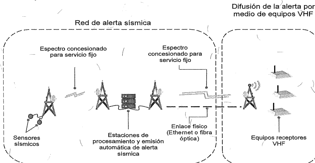
Figura 4. Alternativa de difusión de alerta a equipos receptores en VHF
