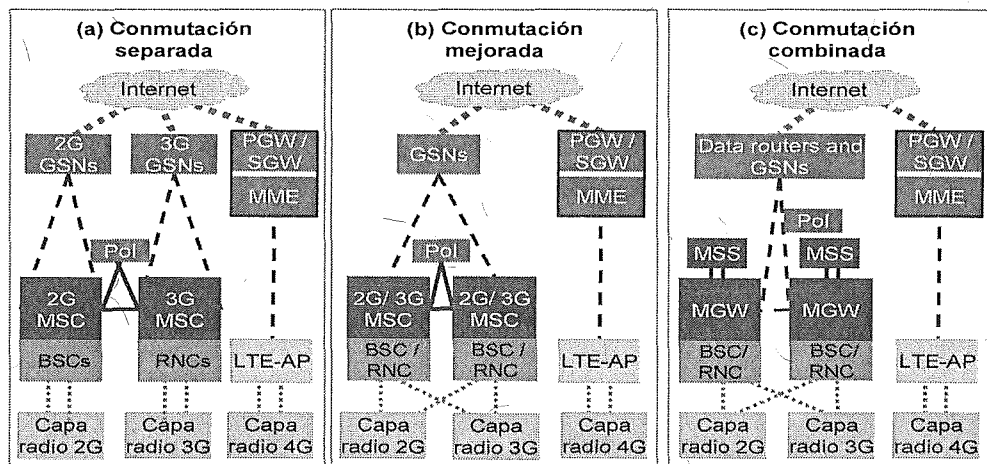
Figura 1. Opciones de arquitectura para el Modelo Móvil.
