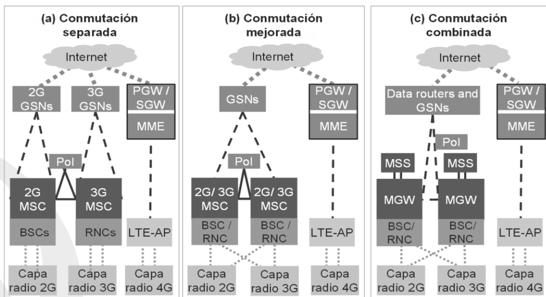
Figura 1. Opciones de arquitectura para el Modelo Móvil.
