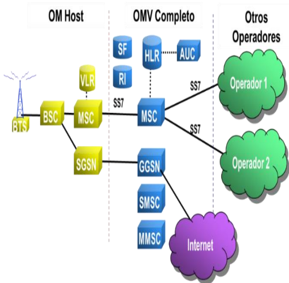
Diagrama 1. Elementos de la infraestructura de la red de un OMV Completo
