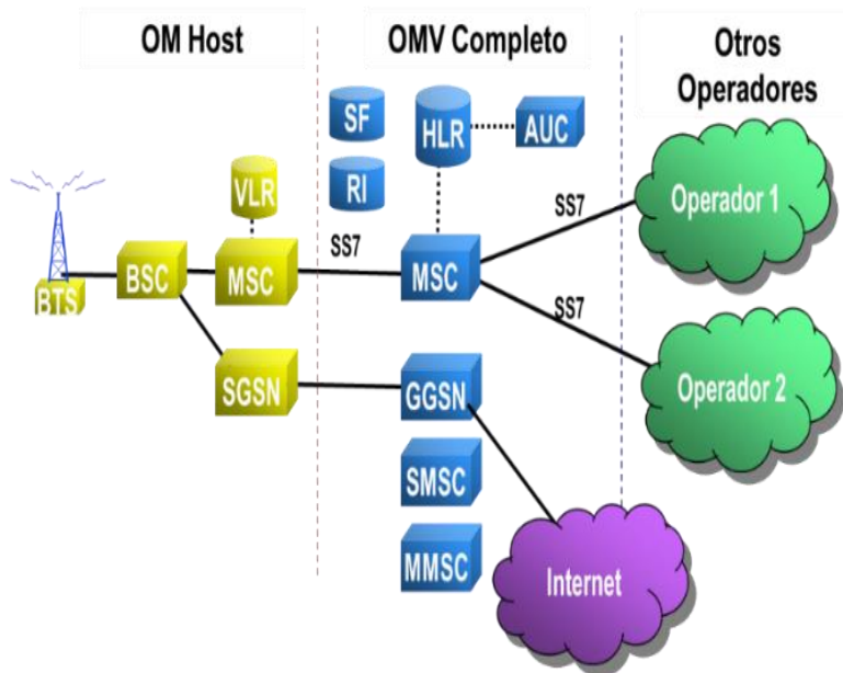
Diagrama 1. Elementos de la infraestructura de la red de un OMV Completo
