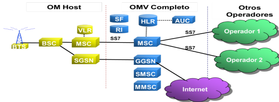
Diagrama 1. Elementos de la infraestructura de la red de un OMV Completo
