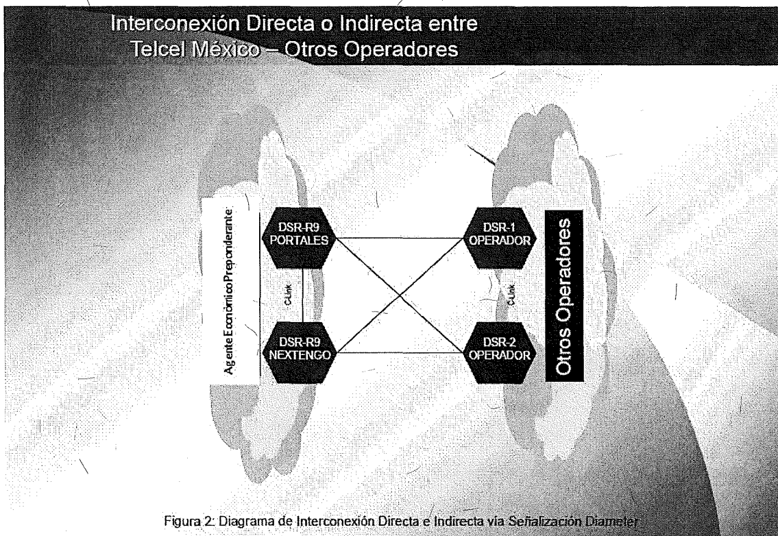
Figura 2: Diagrama de interconexión directa e indirecta vía señalización Diameter
